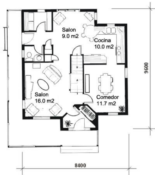
Planta baja
