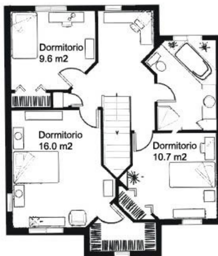
Primera planta
