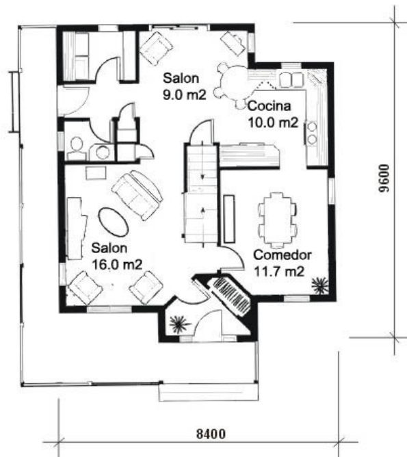
Planta baja
