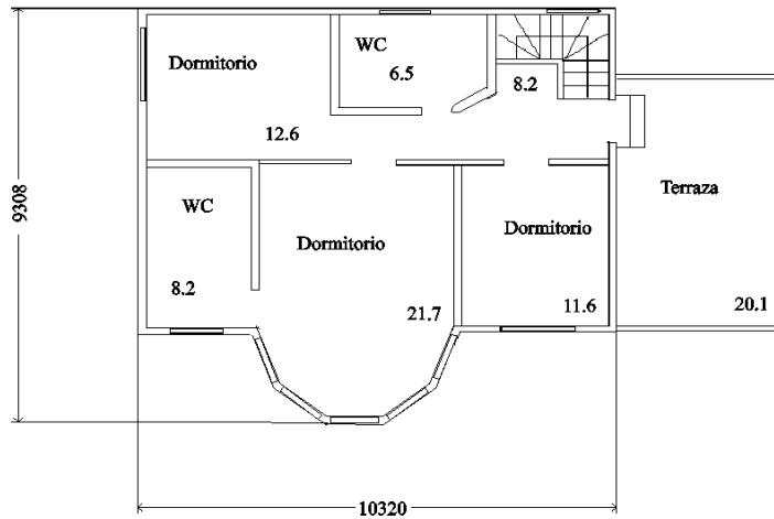
Plano primera planta
