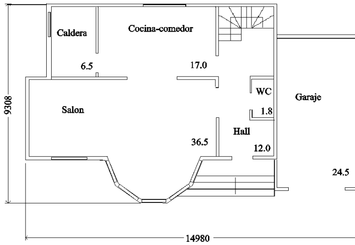
Plano planta baja
